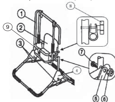
Рисунок 2. Сборка качелей
