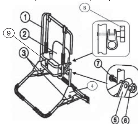
Рисунок 2. Сборка качелей
